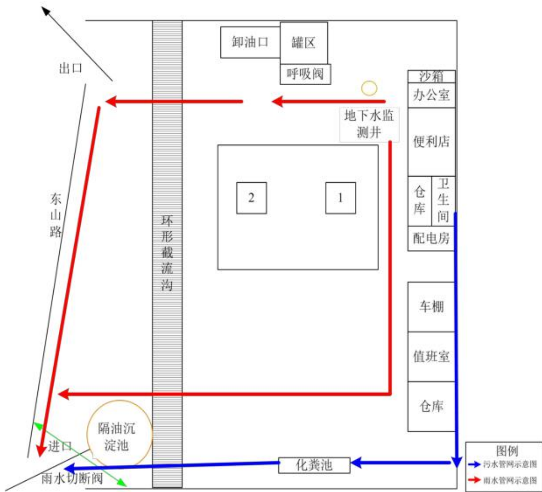
附图 3 项目雨污管网图
