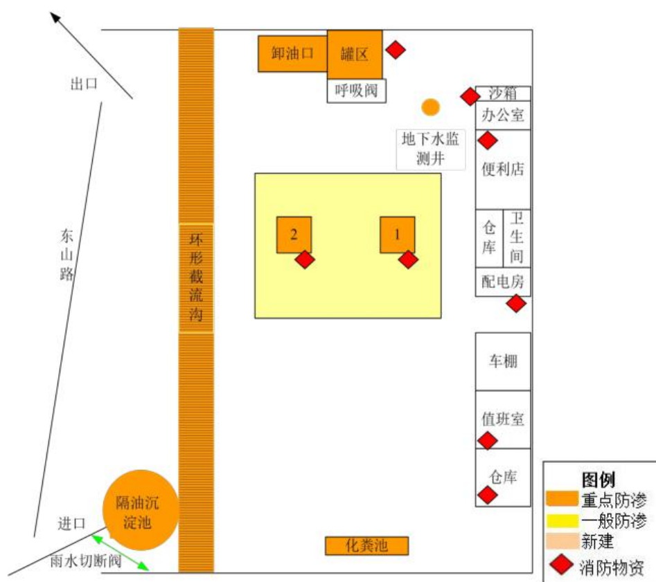
附图 2 项目平面布置图
