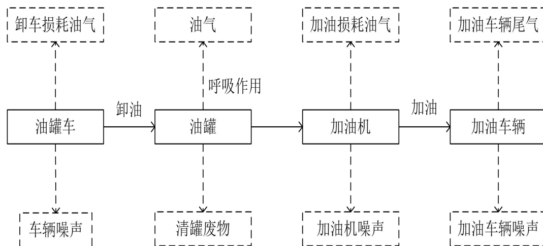
图 2.1-2 柴油加油工艺流程及产污环节图
