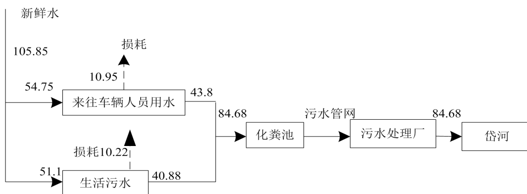
图 2.1-1 项目水量平衡图 (t/a)
