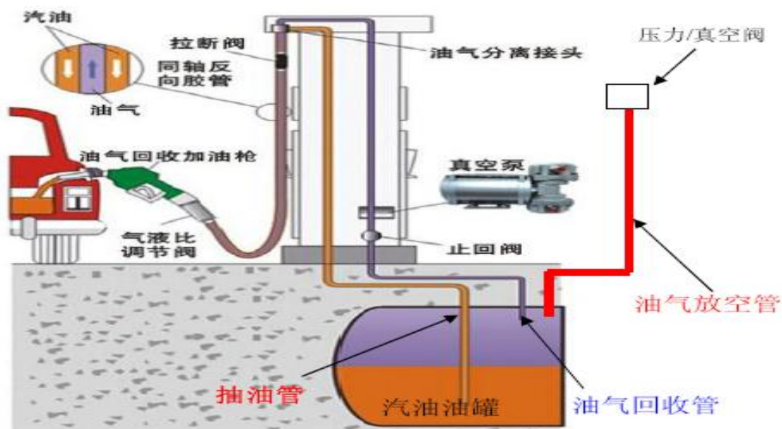
图 2.1-5 二次油气回收系统示意图
