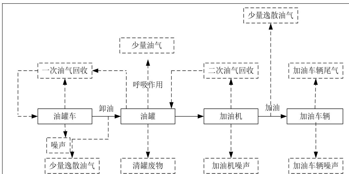
图 2.1-3 油气加油工艺流程及产污环节图
