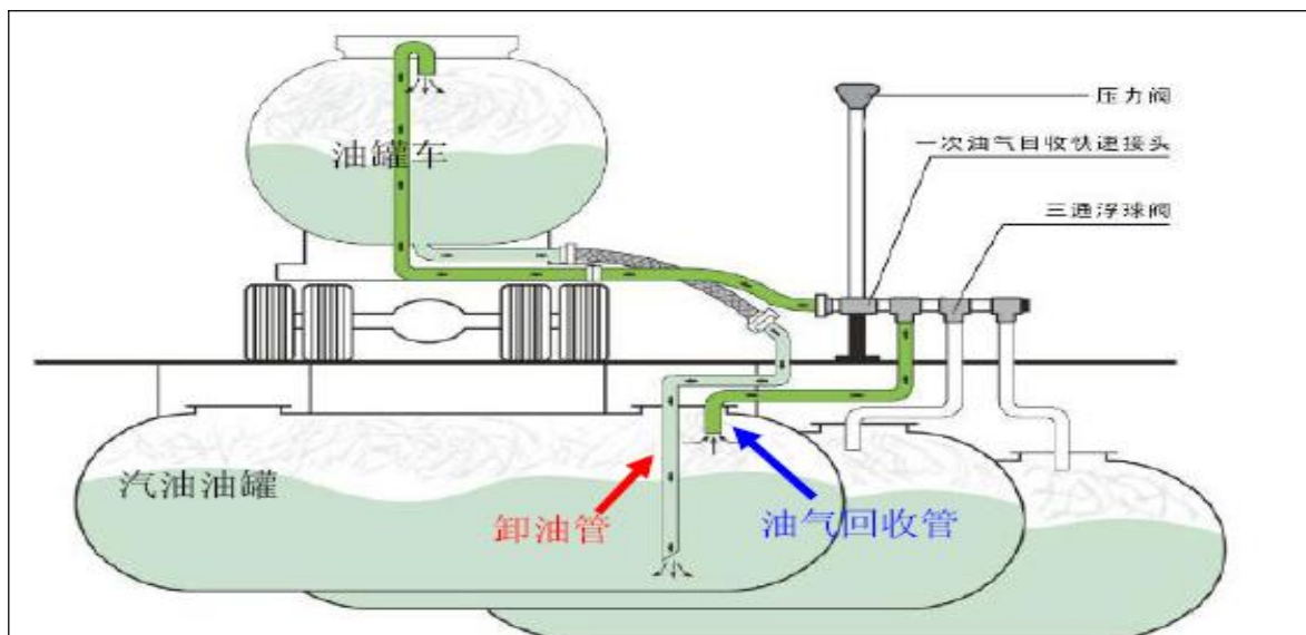
图 2.1-4 一次油气回收系统示意图
